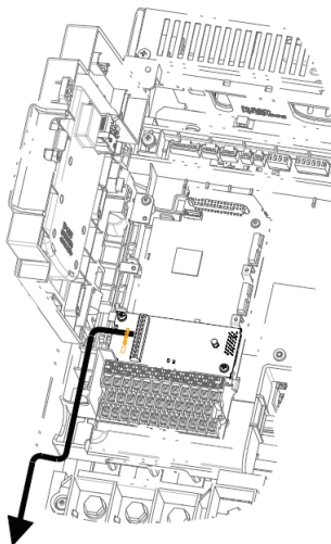
図 4.5 配線例
