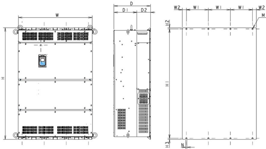
Abbildung 5 Externe Abmessungen des Umrichters (FRN500AQ1S-4□ bis FRN710AQ1S-4□)
