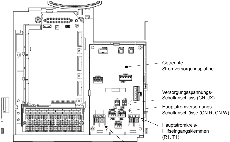
Abbildung 2.5 Anordnung der Schaltanschlüsse (45 kW bis 90 kW)
