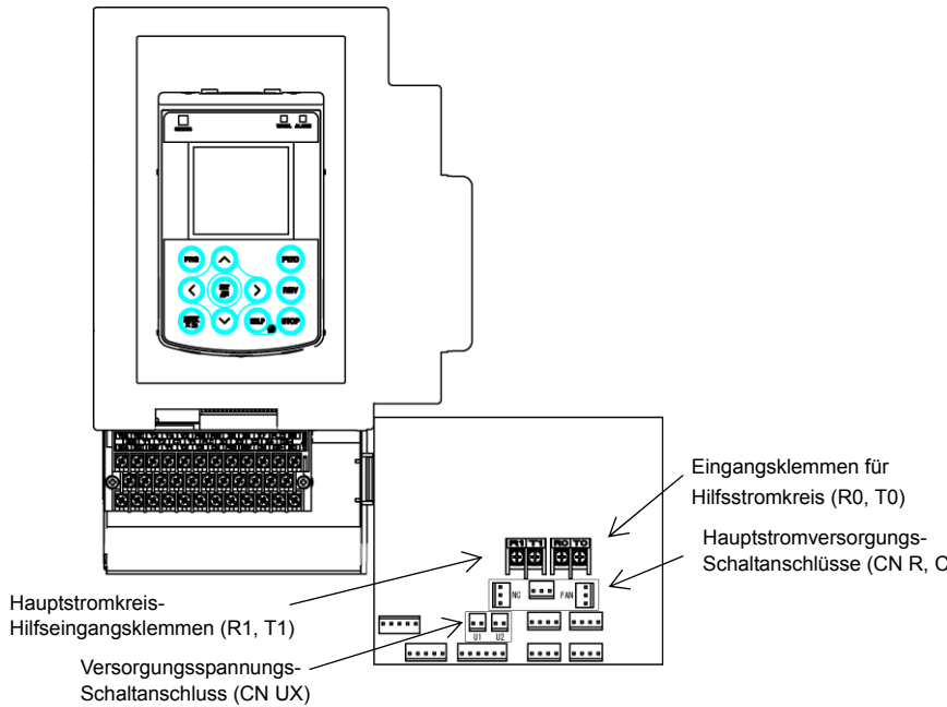
Abbildung 2.7 Anordnung der Schaltanschlüsse (160 kW oder mehr)
