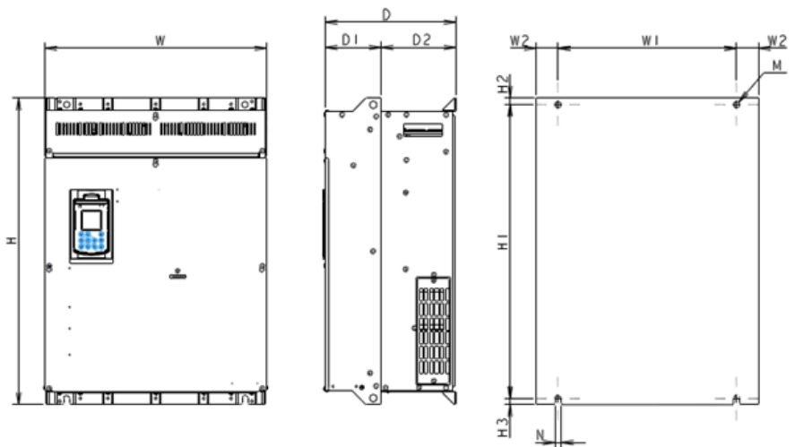
Abbildung 3 Externe Abmessungen des Umrichters (FRN110AQ1S-4□ bis FRN200AQ1S-4□)
