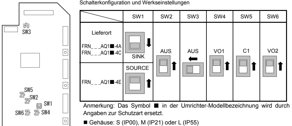
Abbildung 2.9 Anordnung der Schiebeschalter auf der Steuerungsplatine
