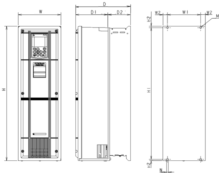
Abbildung 1 Externe Abmessungen des Umrichters (FRN0.75AQ1■-4□ bis FRN37AQ1■-4□)
