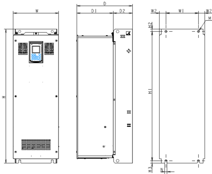
Abbildung 2 Externe Abmessungen des Umrichters (FRN45AQ1■-4□ bis FRN90AQ1■-4□)
